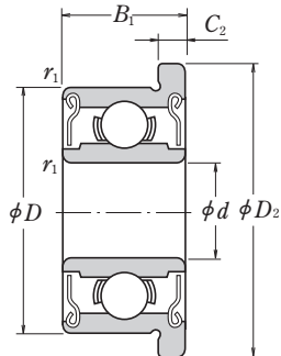
Mit Deckscheiben
