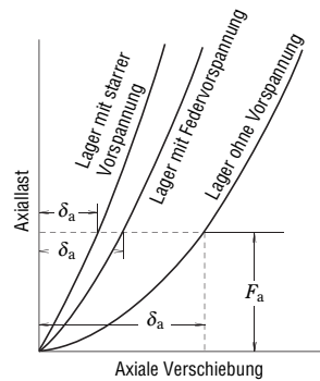
Abb. 10.6 Vergleich von Steifigkeiten und Vorspannmethode
