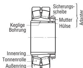
Pendelrollenlager
