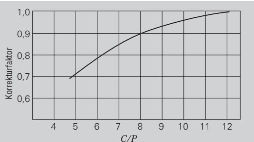
Abb. 6.1 Abhängigkeit des Korrekturfaktors vom Belastungsverhältnis
