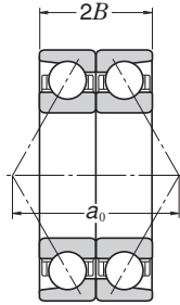
O-Anordnung DB
